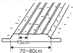
図3 トンネルの被覆
